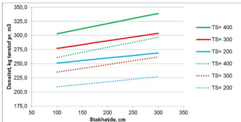
Figur 2. Kg tørstof pr. m 3 som funktion af stakhøjde samt tørstof- (g/kg) og NDF-indhold på 350 (—) eller 440 (•••) g/kg TS.
